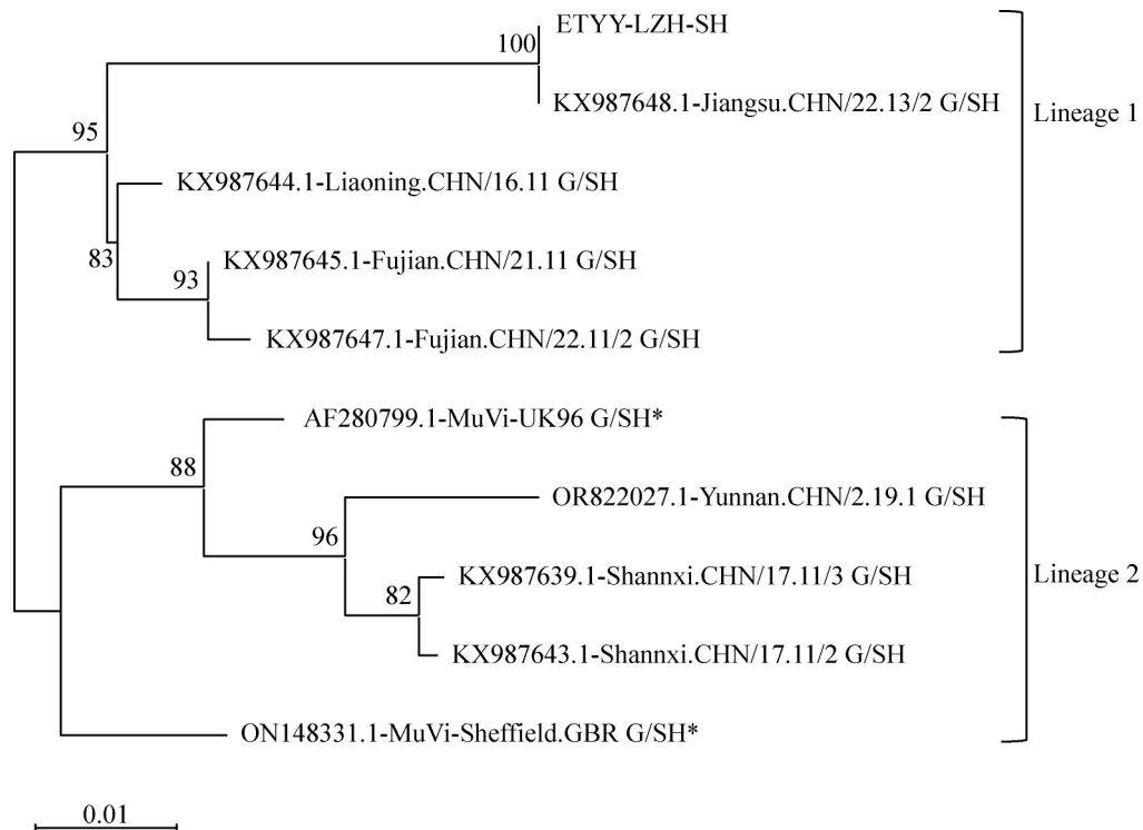
图2 ETYY-LZH株与我国不同地区G基因型毒株基于SH基因的系统发育树构建。同地区SH序列相同仅保留1个毒株进行构建。
