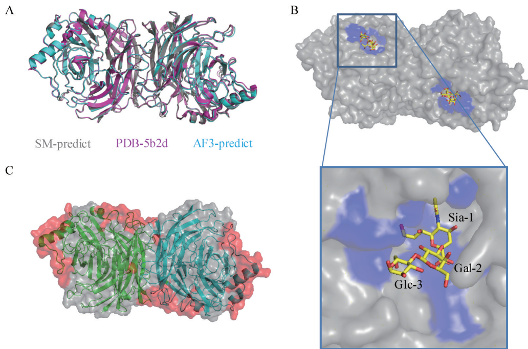
图3 ETYY-LZH株HN蛋白结构分析。 A: HN蛋白的结构预测。ETYY-LZH株的HN蛋白结构采用SWISS-MODEL (SM)和AlphaFold3 (AF3)进行预测, 参考毒株为Hoshino株(PDB: 5b2d, 序列相似性为97.1%), 预测结构与参考毒株C \alpha 的RMSD分别为0.114 Å和0.292 Å。B: HN蛋白与3'-SL的复合物结构预测。图中紫色区域为SWISS-MODEL预测结构识别3'-SL的结合表位, 具体为aa 180、407、422、512、540、561、204、242、254、323、369、476, 其中Sia为唾液酸、Gal为半乳糖、Glc为N-乙酰葡萄糖。C: HN蛋白的B细胞表位分布。图中红色区域为B细胞表位, 分别为aa 113-130 (结构中未展示)、aa 199-207、aa 220-240 (结构内部)、aa 261-266、aa 327-363、aa 375-403、aa 440-443、aa 533 [9] 。
